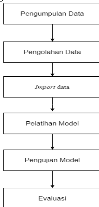
Gambar 1. Kerangka penelitian
