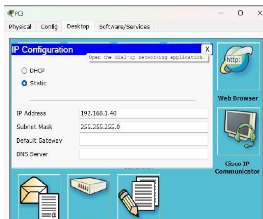
Gambar 5. IP Address Pada PC3
