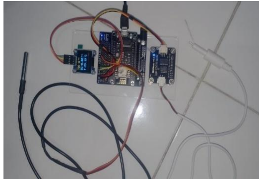
Gambar 2. Rancangan Keseluruhan Perangkat Keras
