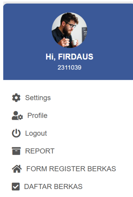
Gambar 5. Halaman Beranda
